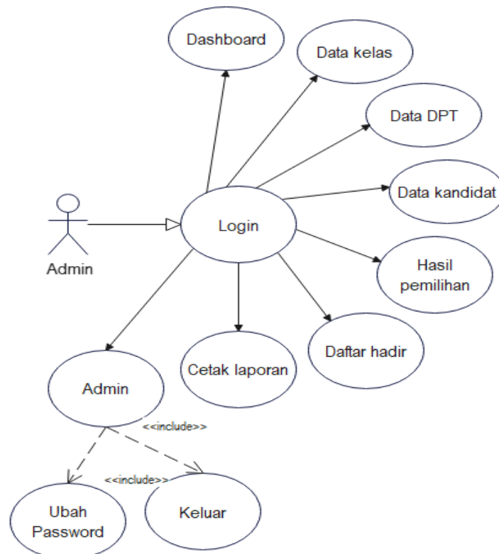
Gambar 2. Use Case Diagram Admin, yang mencakup fungsionalitas inti seperti mengelola data kelas, data DPT, data kandidat, memantau daftar hadir, dan mencetak laporan resmi
